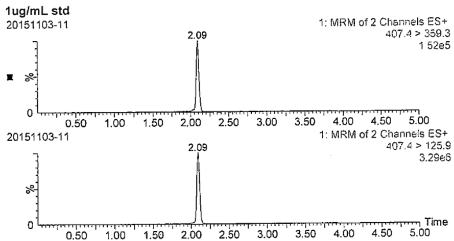
林可霉素对照溶液得到的特征离子质量色谱图
